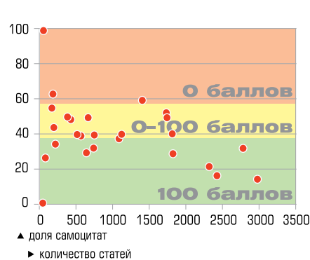
Доля самоцитат у университетов. Физика и астрономия
