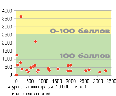
Концентрация статей у университетов. Физика и астрономия
